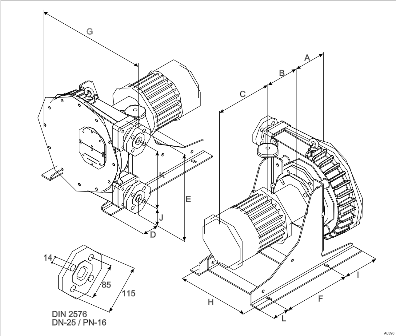
Fig. 17: Dimensions DFDa 025
