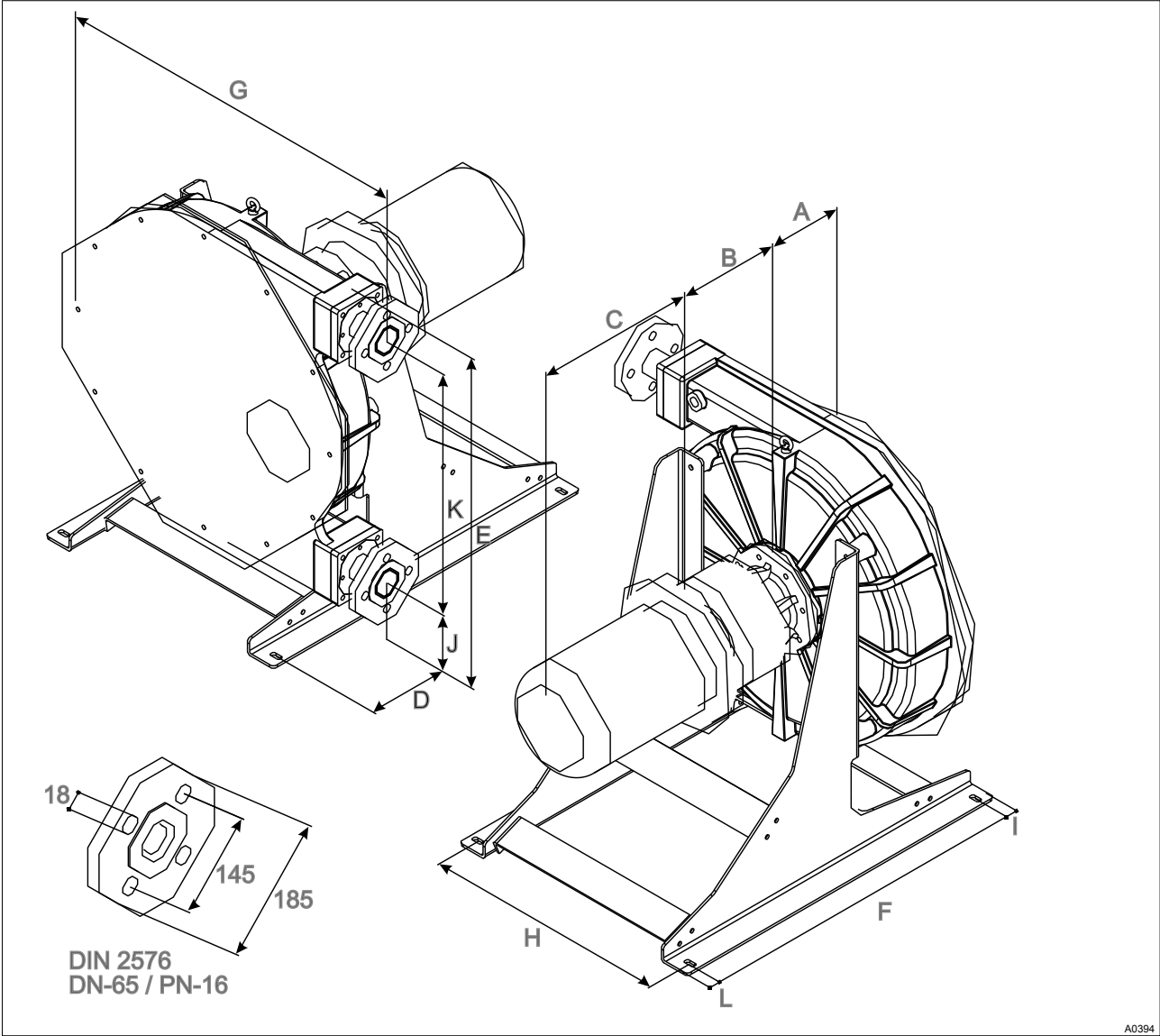
Fig. 21: Dimensions DFDa 070
