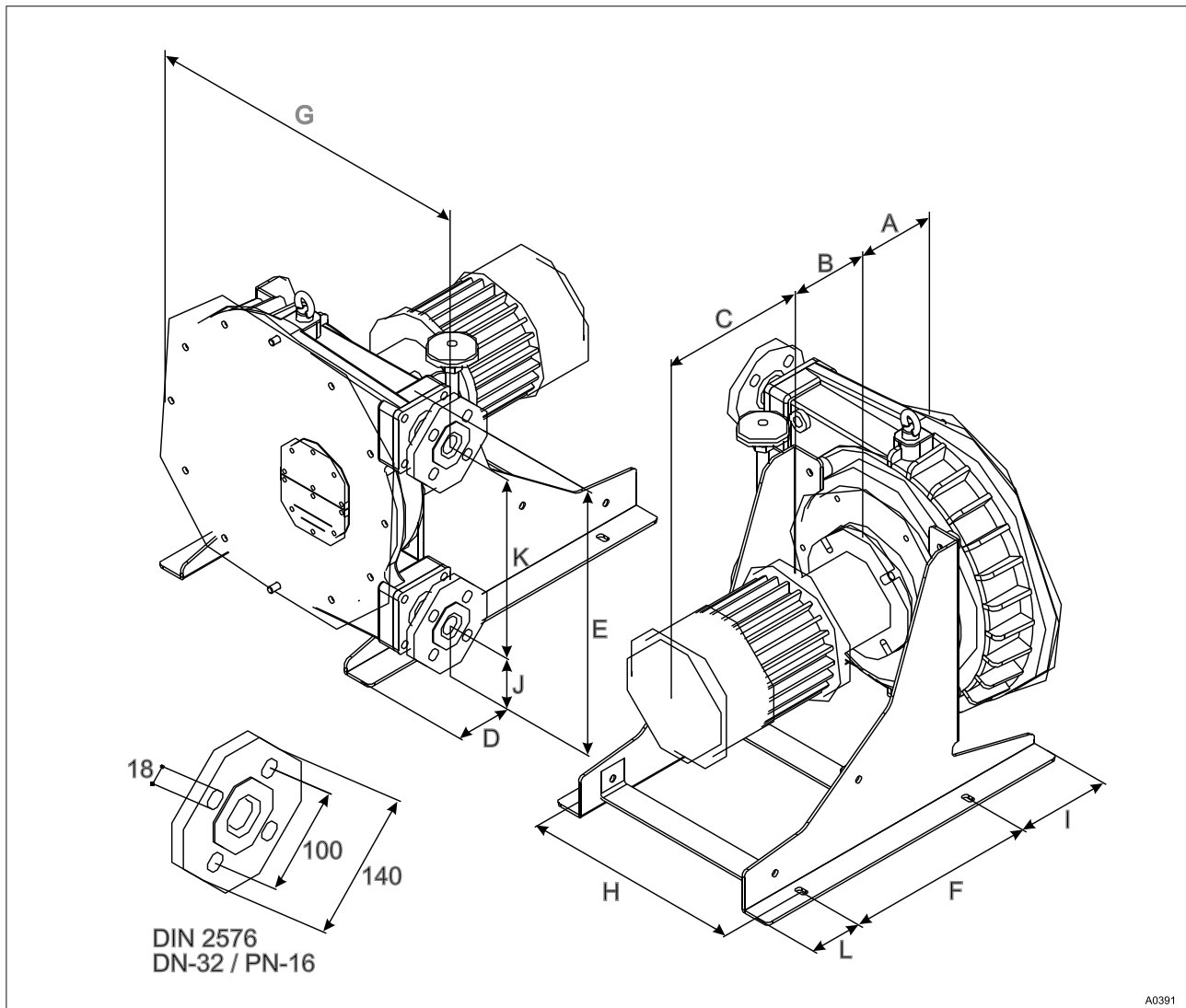
Fig. 18: Dimensions DFDa 032
