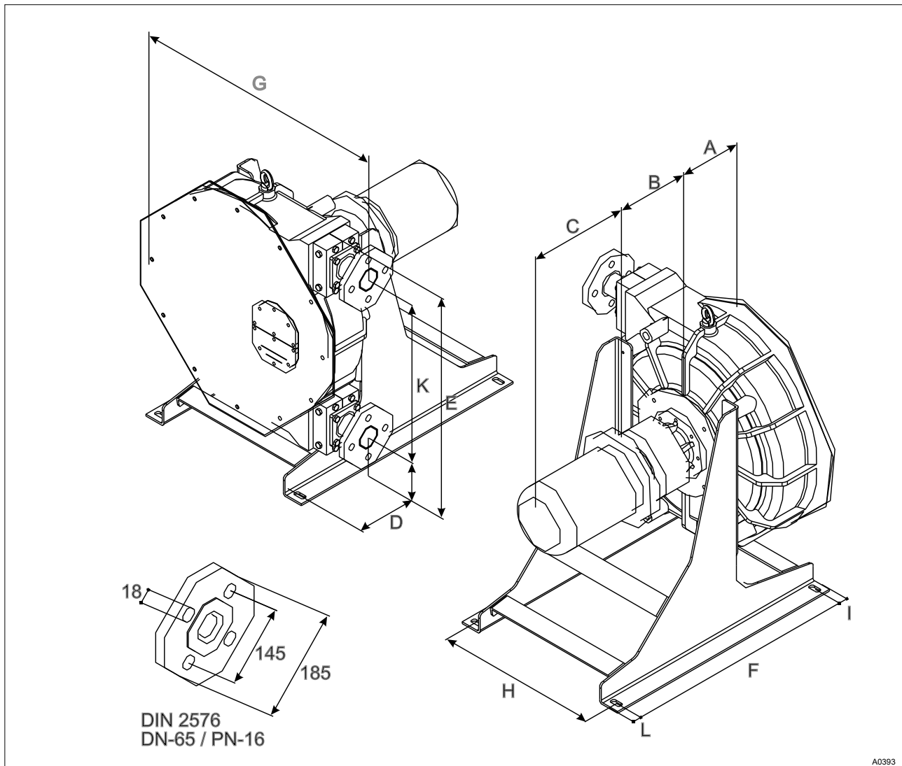
Fig. 20: Dimensions DFDa 060
