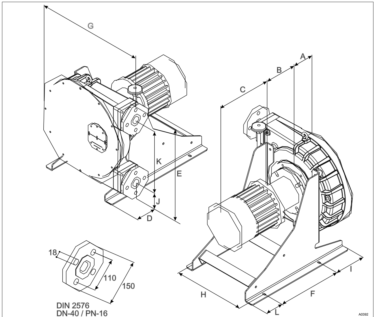
Fig. 19: Dimensions DFDa 040
